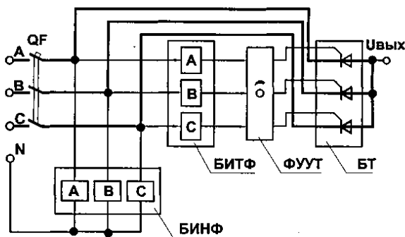
ПРИЛОЖЕНИЕ А Функциональная схема устройства дожига УД-300
